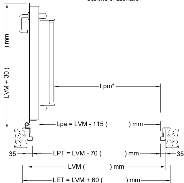
Sezione Orizzontale
