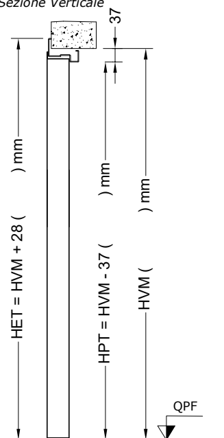
Sezione Verticale
