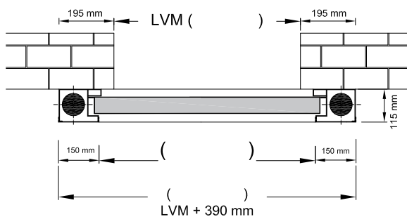
SEZIONE ORIZZONTALE
