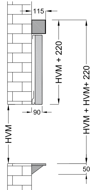
Sezione Verticale
