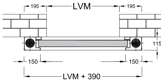
Sezione Orizzontale
