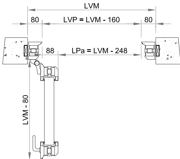
Sezione Orizzontale
